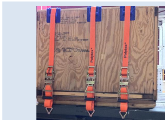
Arrimage par frottement / par le dessus
